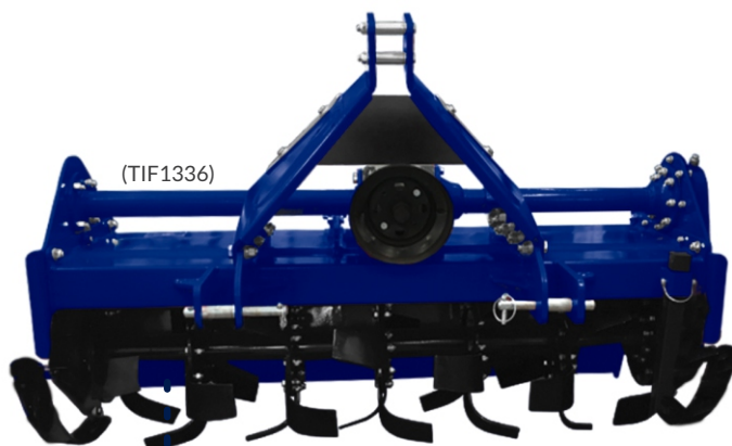
q Patines laterales para ajuste de profundidad
